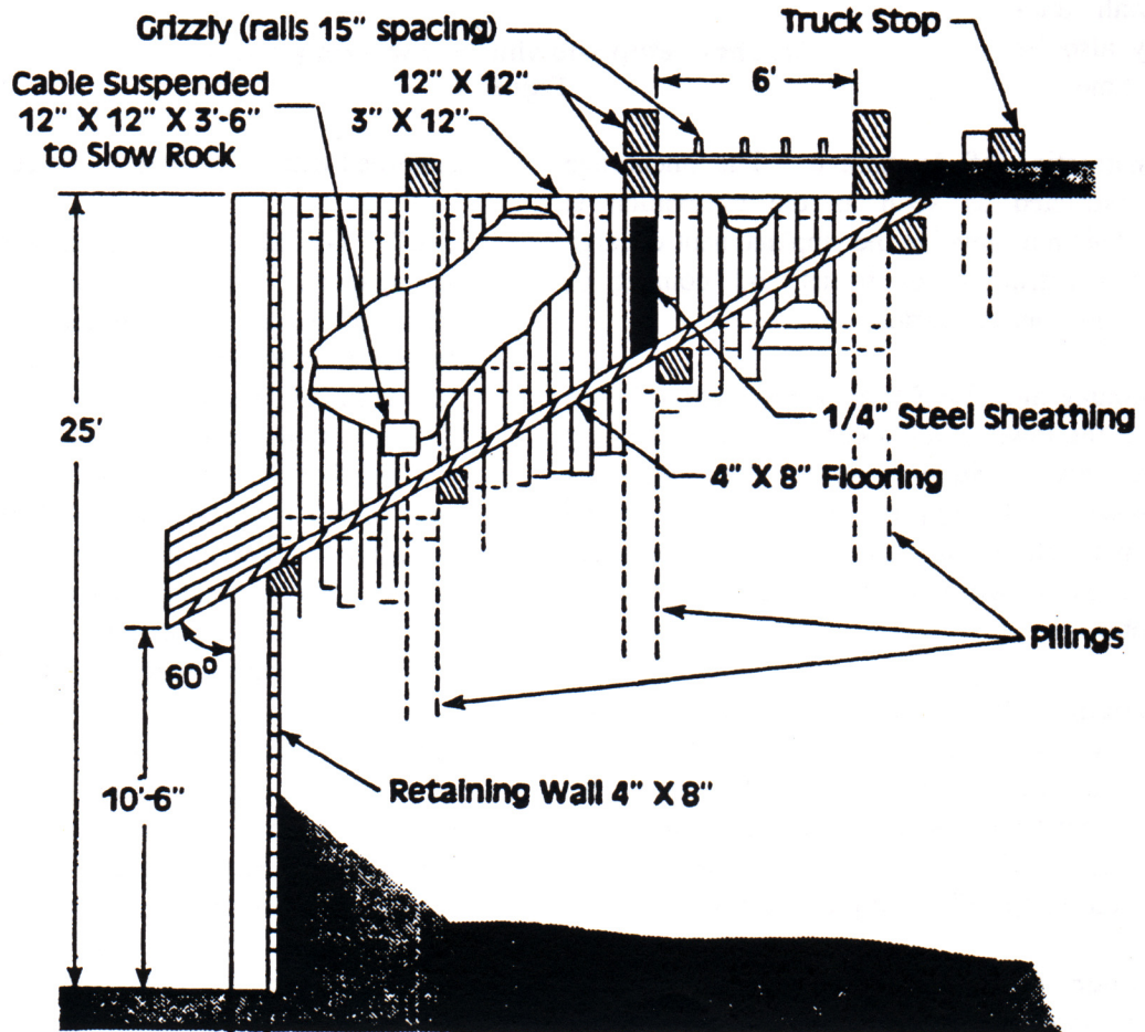
SECTION A-A
